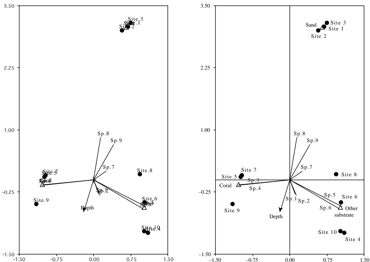
Figure 1 Diagramme de double projection. À gauche, le diagramme produit par le Progiciel R v.4. À droite, le diagramme retouché à l'aide d'un programme de dessin.
